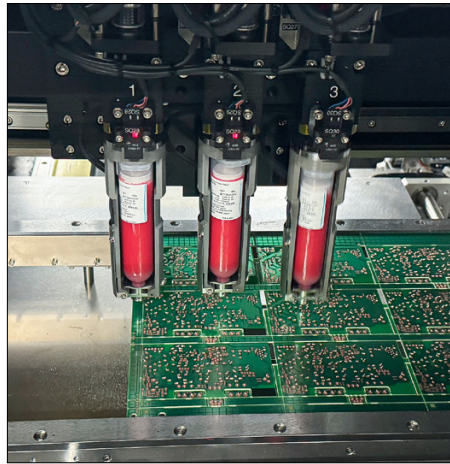
Der schnellen Bewegungen der Maschine können das Auge und selbst eine Kamera kaum folgen.
