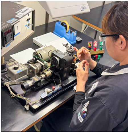
Eine Mitarbeiterin beim Bau eines Denon DL-103, genauer gesagt: dem Wickeln der Spule.
